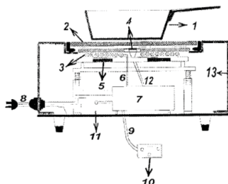
Figura 1. Estructura de la cocina de inducción.
