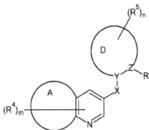
fórmula (I)
