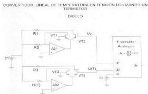
Figura 1. Convertidor de temperatura en tensión utilizando termistor
