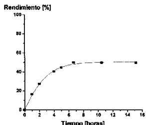
Fig. 1 Curva de rendimiento para el copolímero de 22.2 % molar de ácido acrílico.
